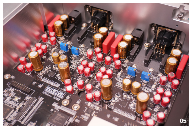
04. 內部02： A15對於電源供應也是非常講究，內部以四顆獨立的屏蔽環形變壓器做區塊的獨立供電，包括「數位電路」、「伺服器電路」，以及「兩只DAC電路」。機內同時可見原廠嚴選的UPS超級電容，電源設計相當豪華。 05. 內部03： A15在DAC部分採用兩只AKM4490晶片達到Dual Mono架構。最高可解碼PCM 32Bit/768kHz、DSD512，以及MQA Full-Decoder，夠讓您用上好幾年不用換機。
